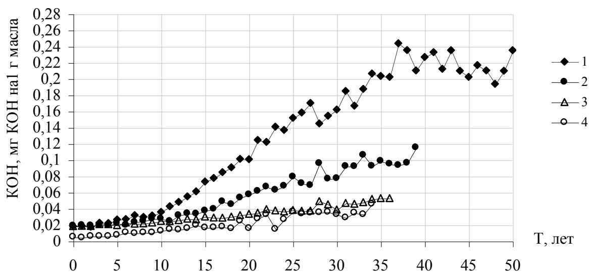
Рисунок 5 – Зависимость кислотного числа трансформаторного масла от времени эксплуатации для массивов однородных данных, квантованных с шагом 1 год 1 – массив M_1 ; 2 – массив M_2 ; 3 – массив M_3 ; 4 – массив M_4
